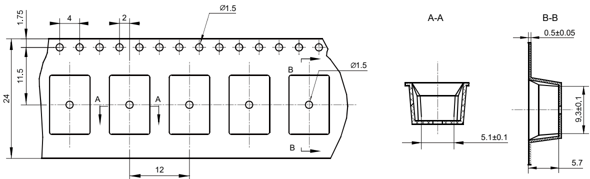
载带外形图
